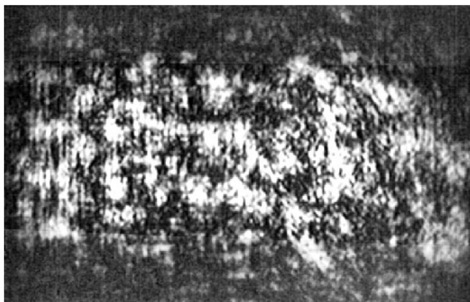
Пучок, прошедший через записанную голограмму
